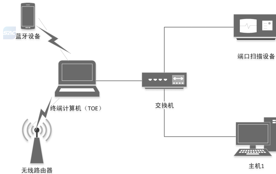
图 1 测试环境图
